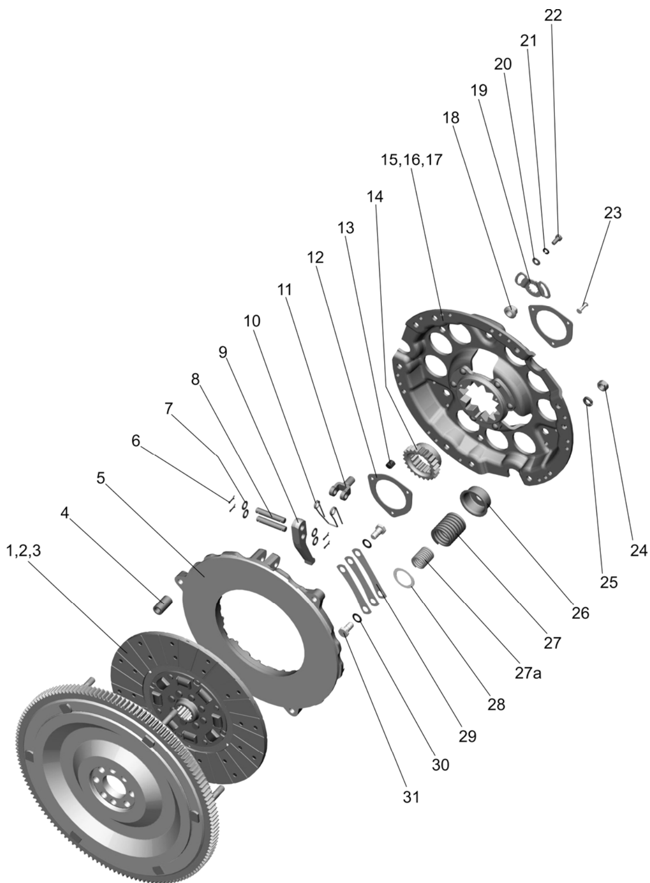
Рис.16.1. Установка сцепления 240-1005009-03
