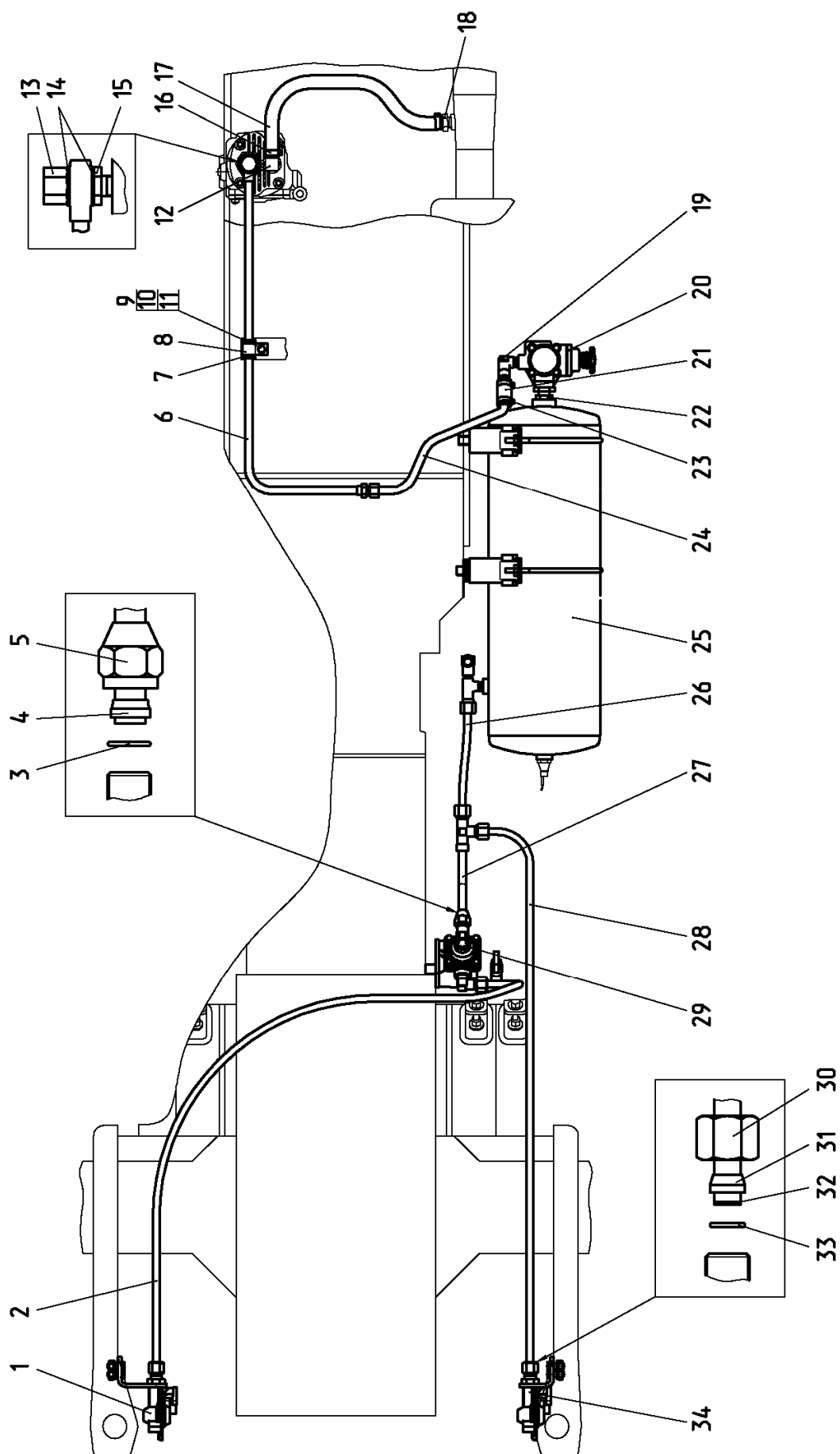
Рис.35.7 Пневмопривод
