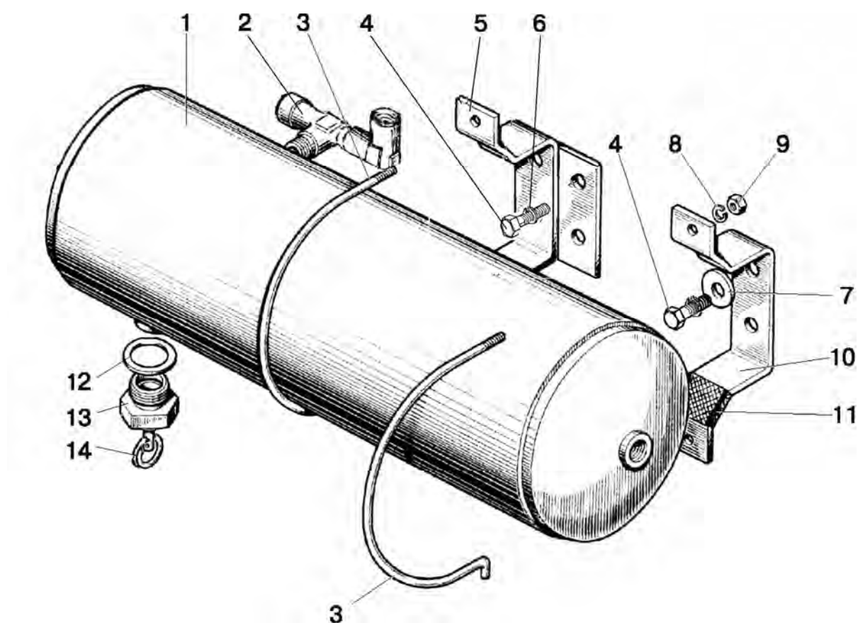
Рис. 35.8. Баллон
