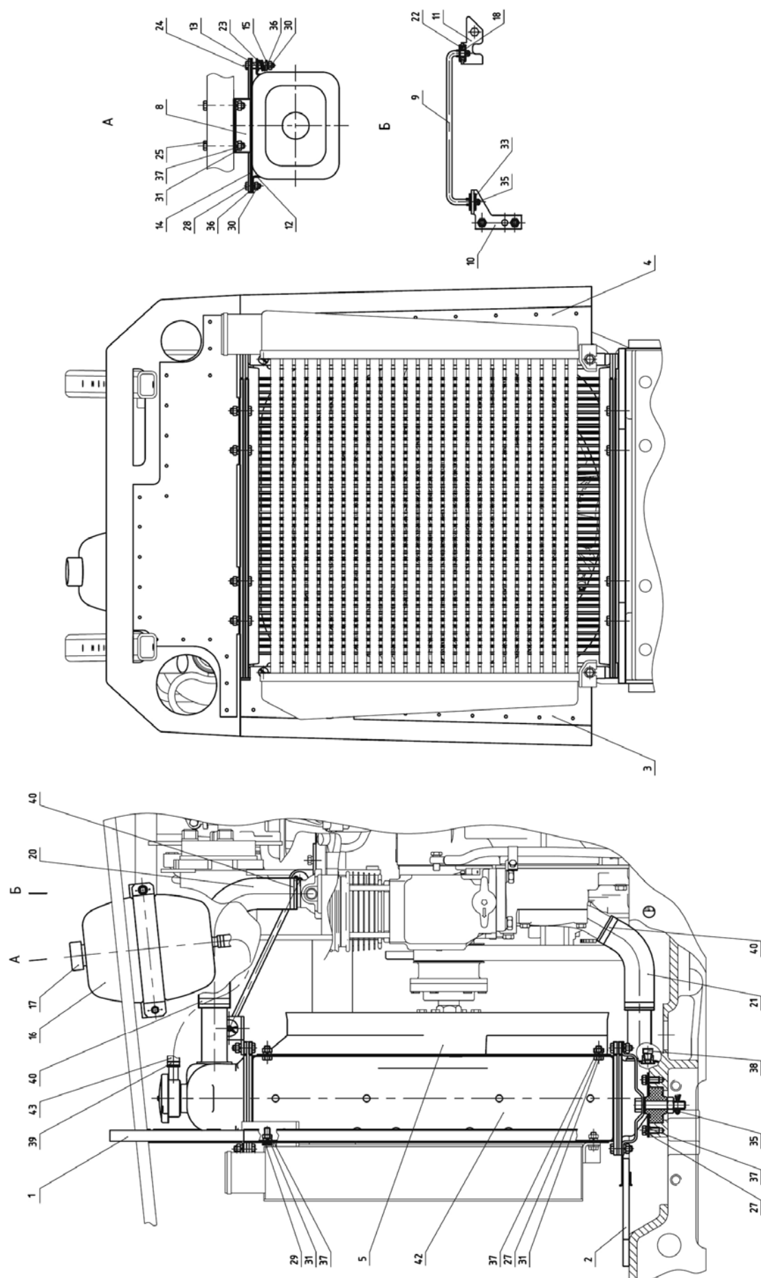
Рис.13.1 Блок охлаждения
