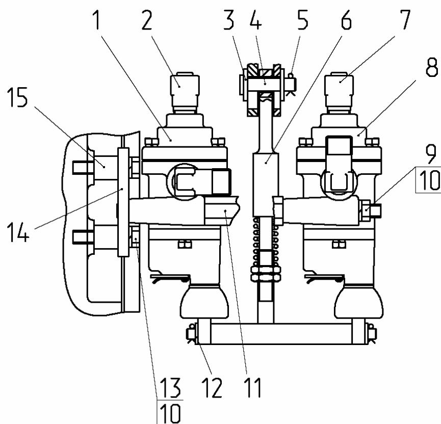
Рис.35.12 Кран тормозной
