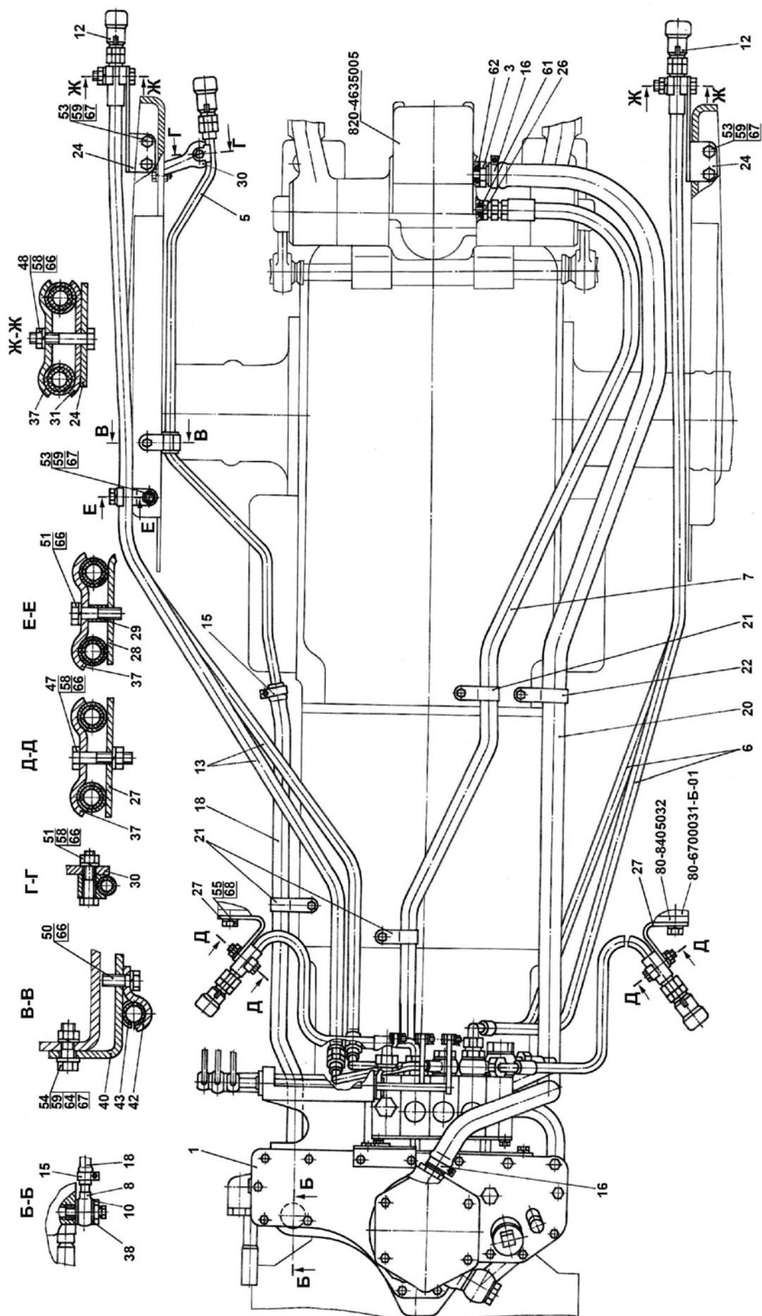
Рис.46.6 Гидросистема Р1221-4600010
