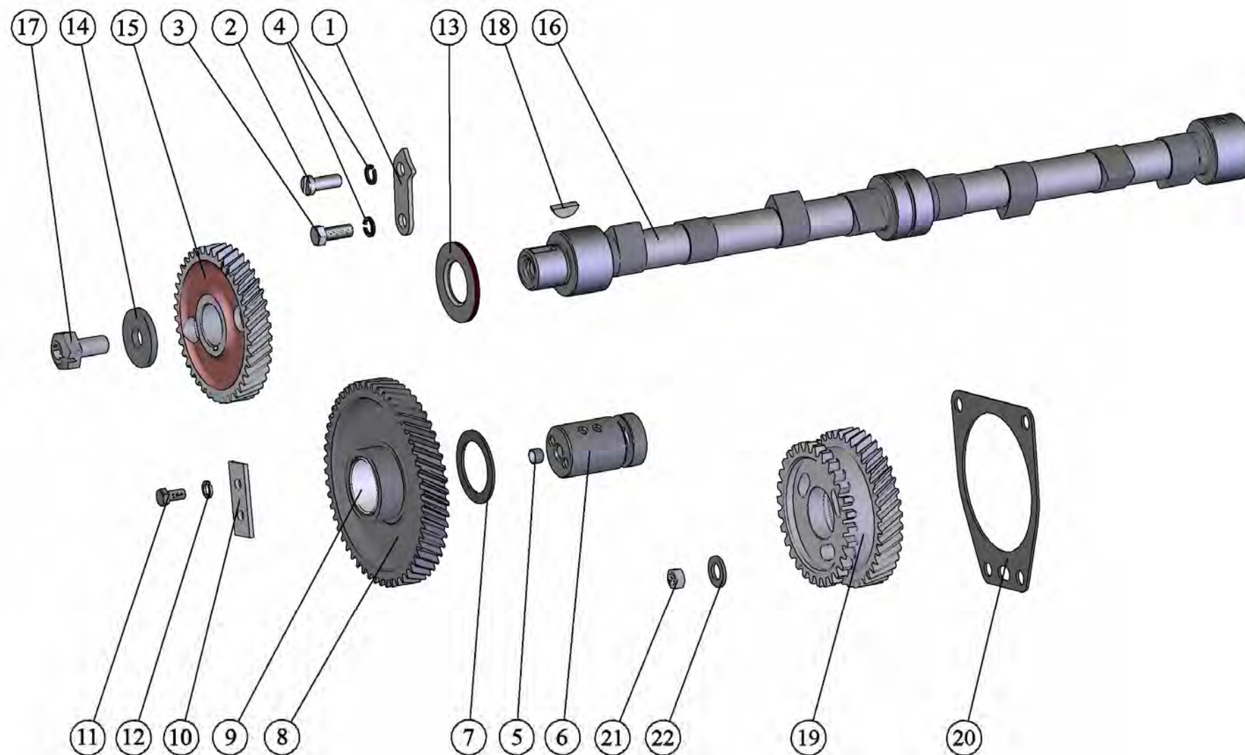
Рис. 4 Распределительный механизм.
