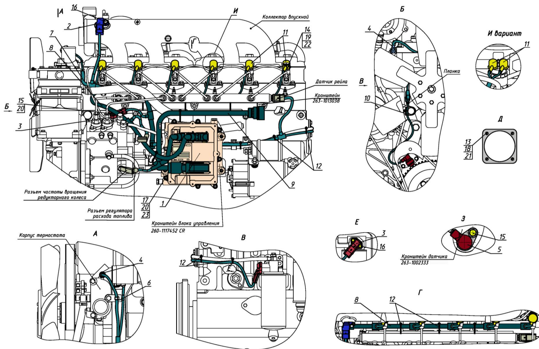
Рис. 23 Электронный блок управления. Установка электрооборудования.
