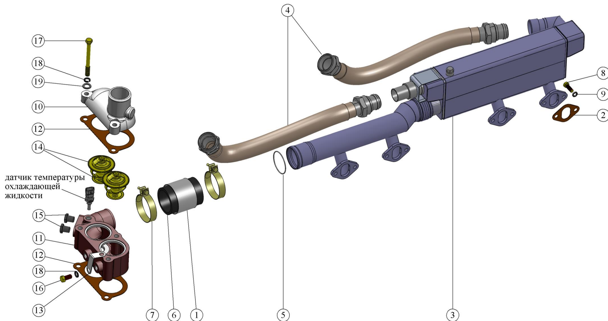
Рис. 11 Установка рециркуляции отработавших газов. Корпус термостатов.
