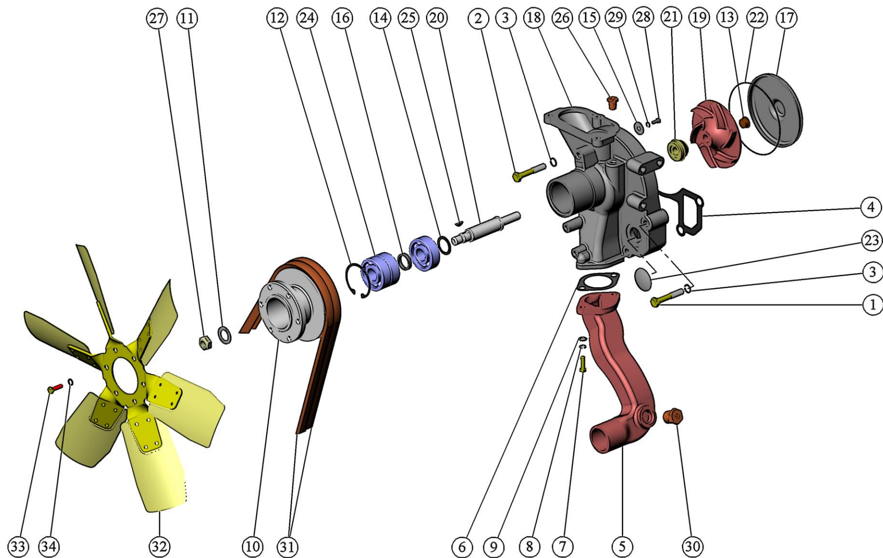
Рис. 12 Установка насоса водяного. Установка вентилятора.
