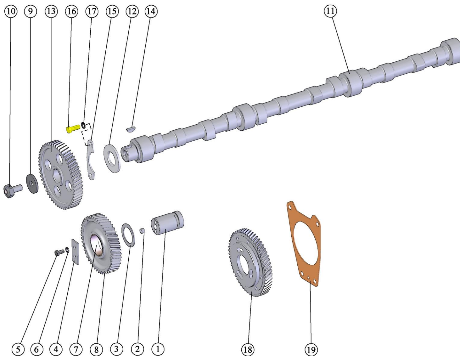
Рис. 5 Распределительный механизм.
