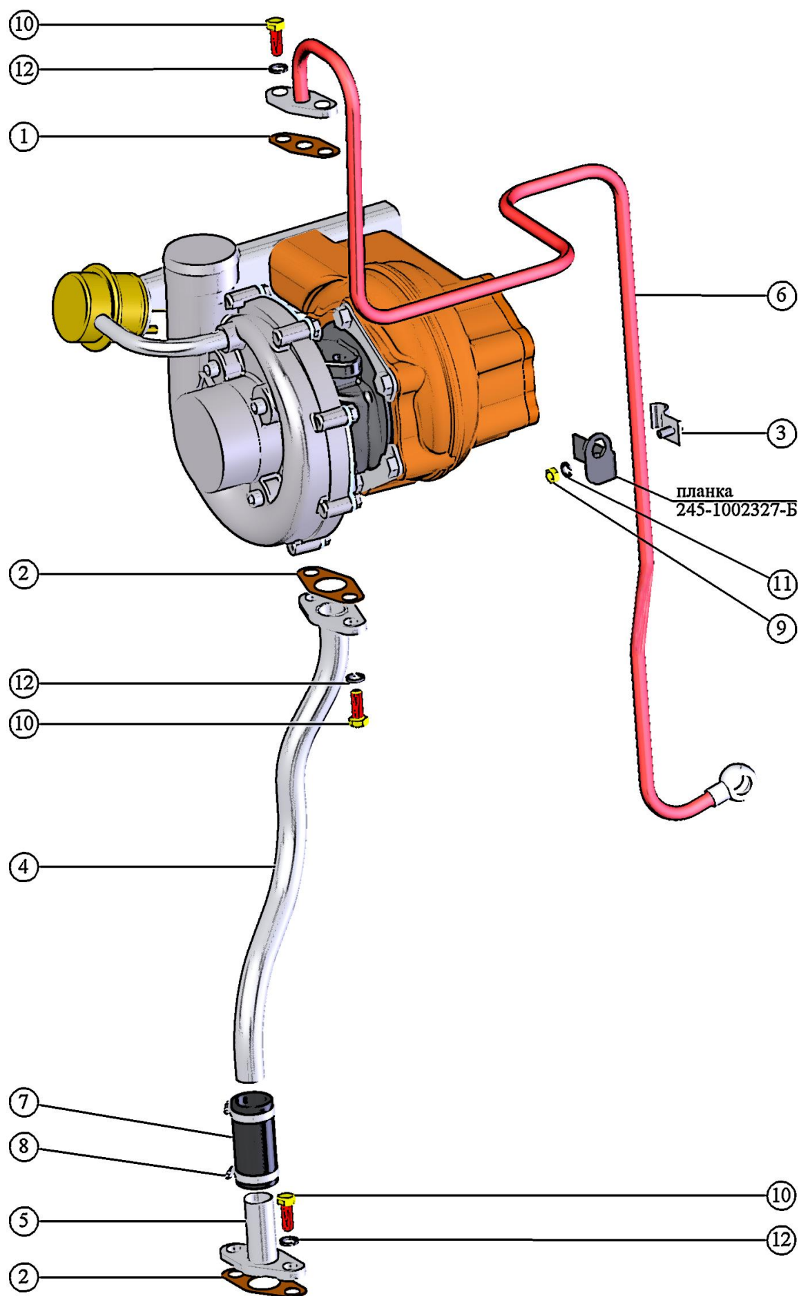
Рис. 19 Маслопроводы турбокомпрессора.
