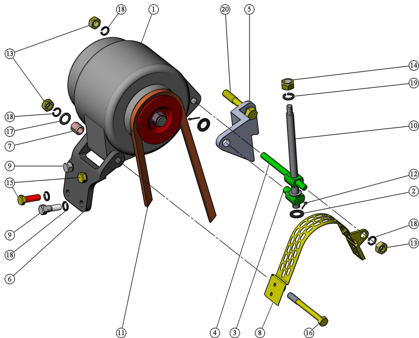
Рис. 24 Установка генератора.
