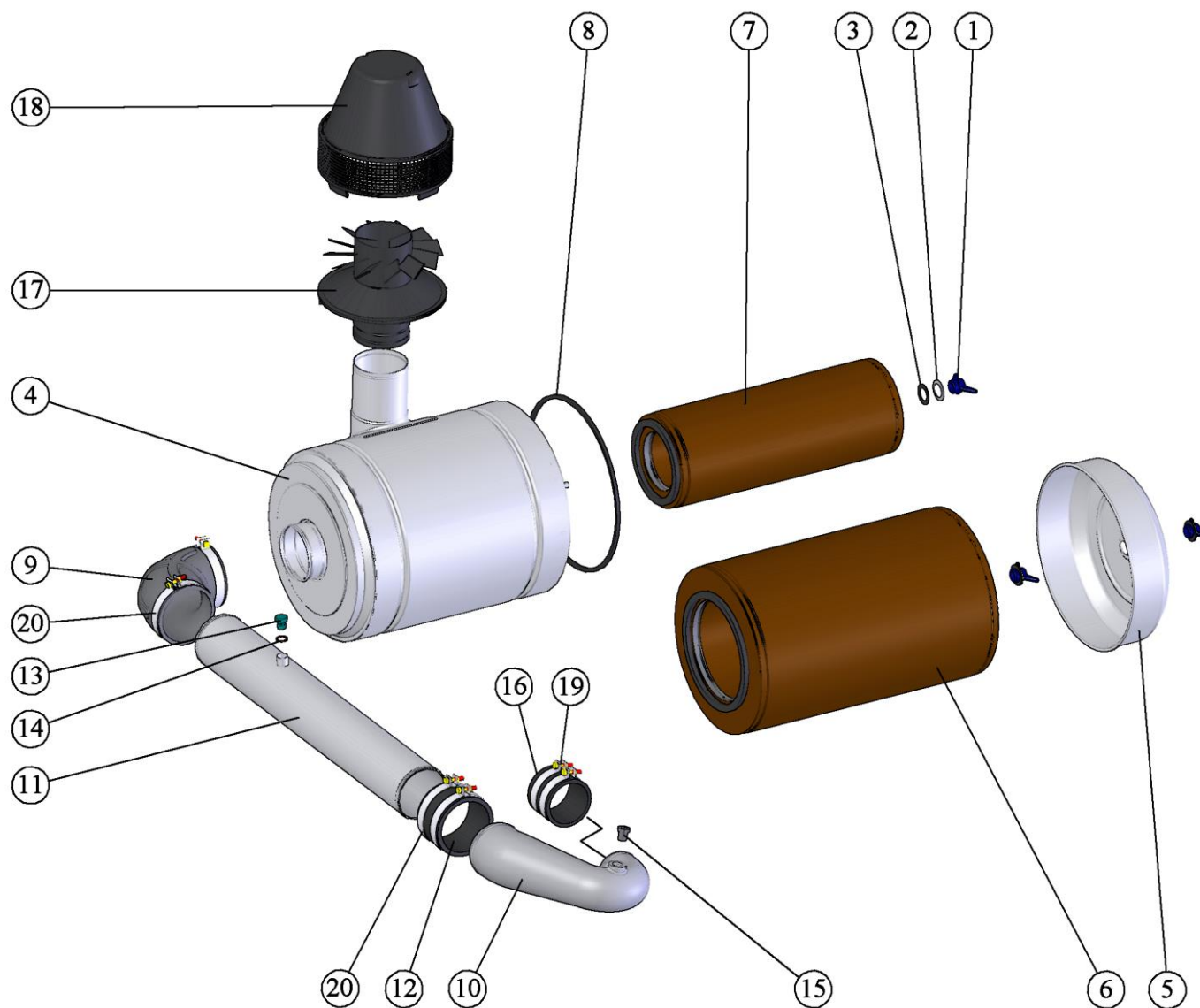
Рис. 25 Воздухоочиститель.
