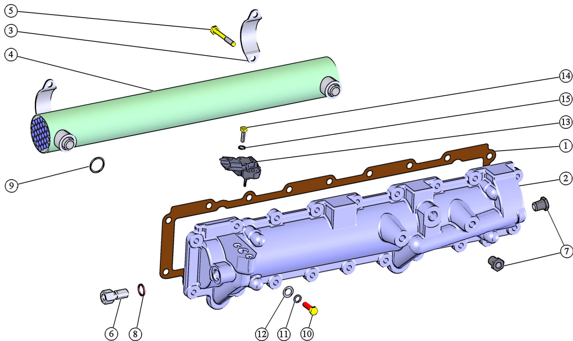
Рис. 16 Установка теплообменника.
