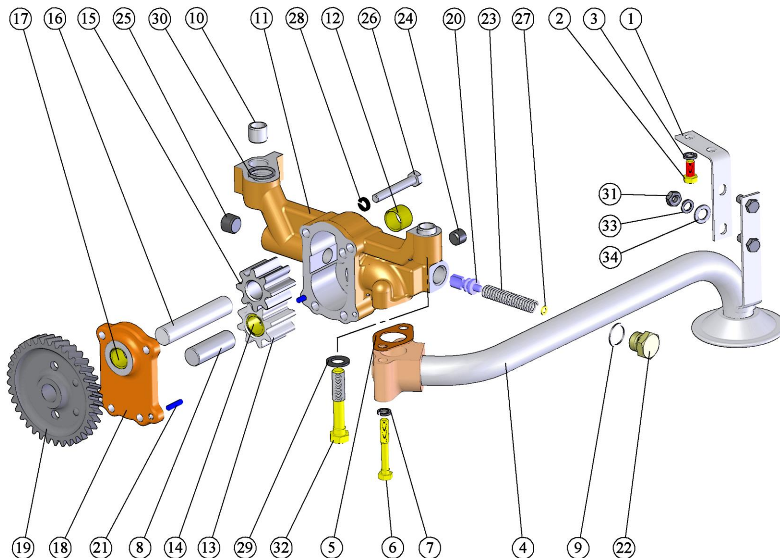
Рис. 15 Установка насоса масляного.
